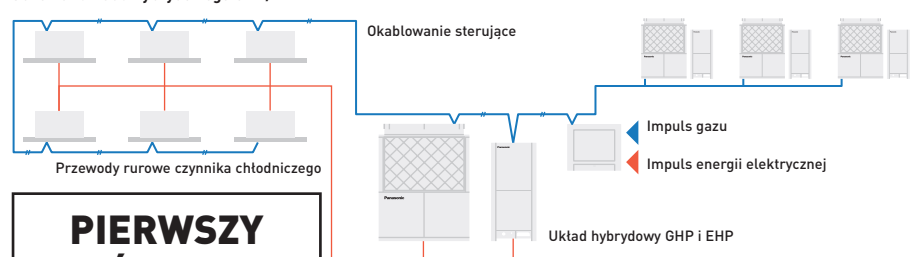
Schemat układu hybrydowego GHP/EHP
