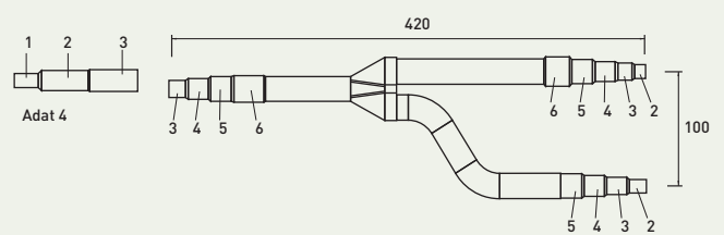
Rura czynnika ciekłego
