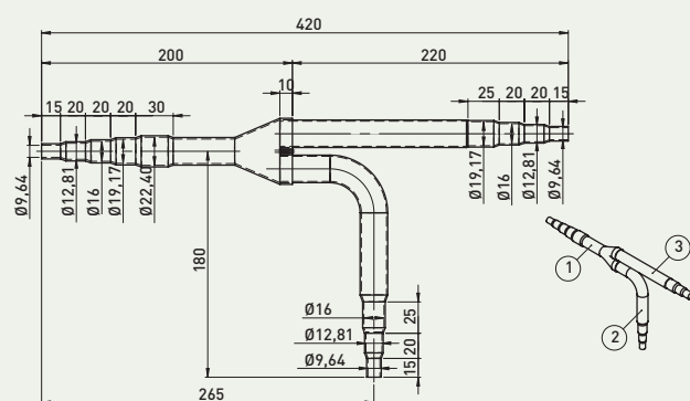
Rura czynnika ciekłego
